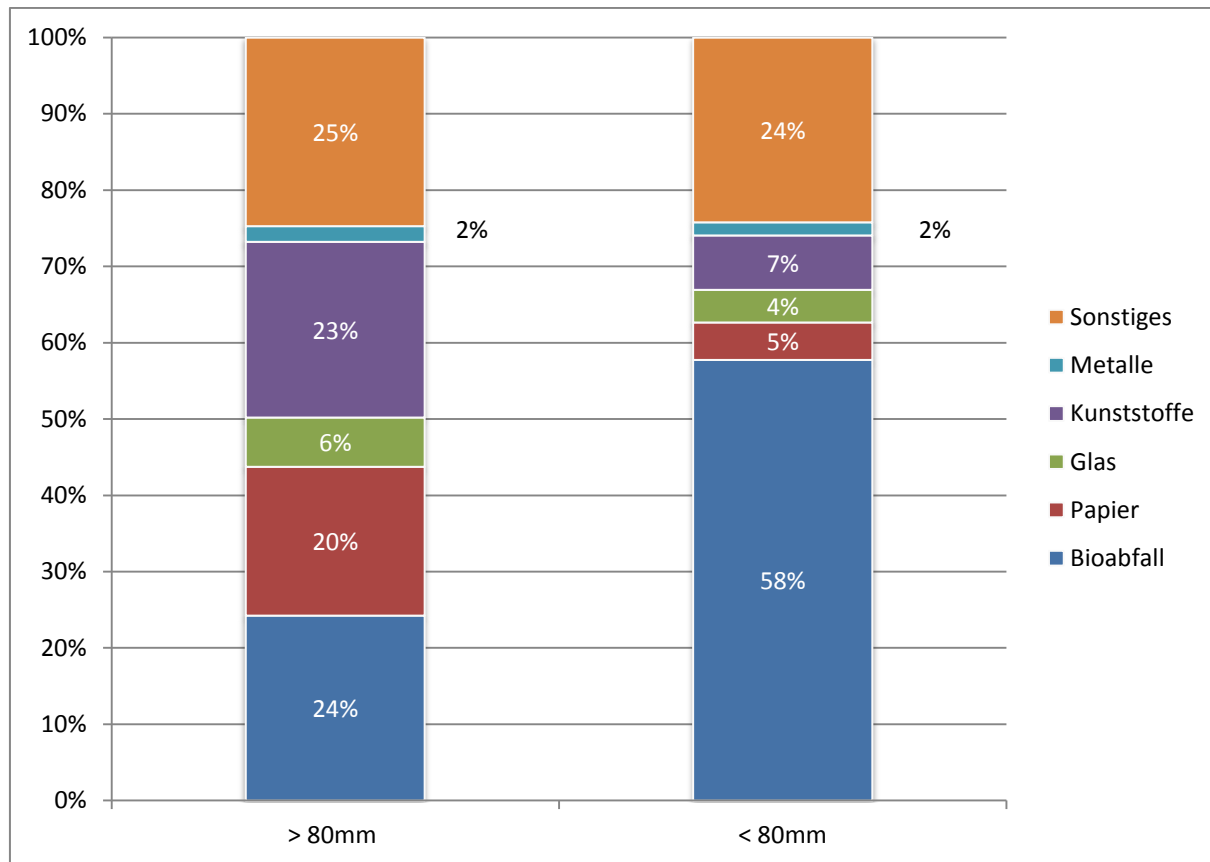
Abbildung 3-32: Stoffliche Zusammensetzung der Kornfraktionen <80 mm und >80 mm
