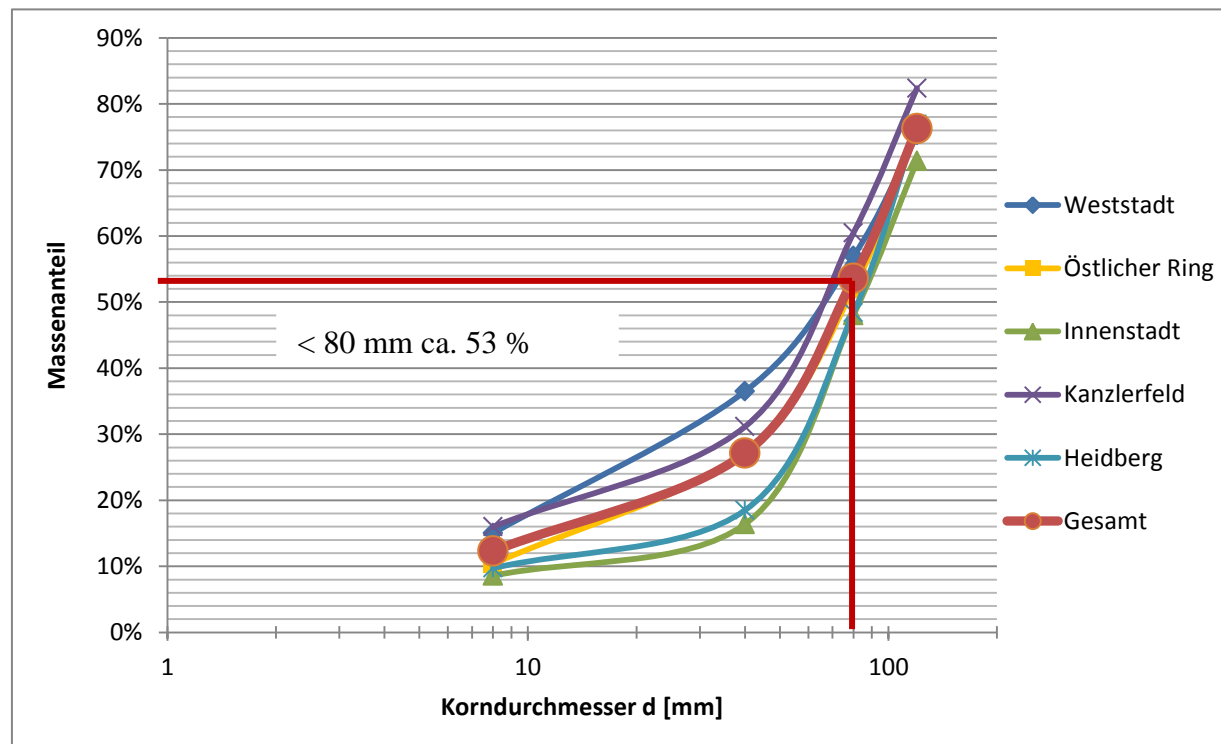
Abbildung 3-31: Sieblinien der einzelnen UG im Stadtgebiet Braunschweig
