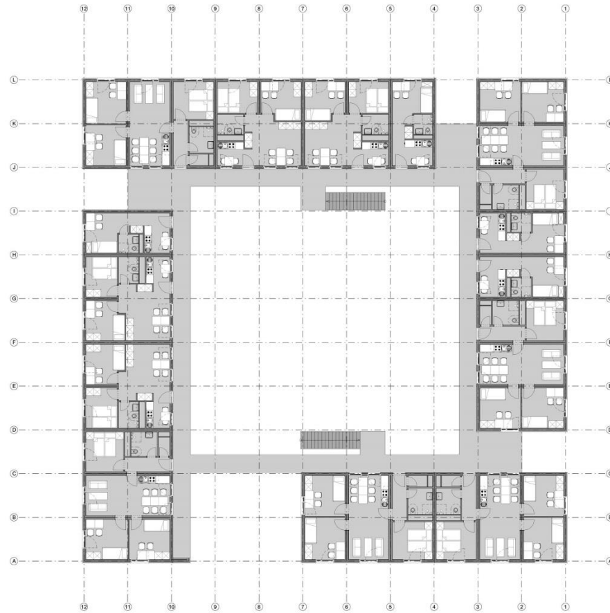
Grundriss Obergeschoss
