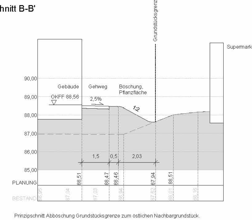
Schnitt B-B'
