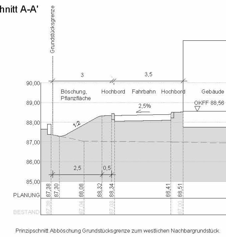
Schnitt A-A'
