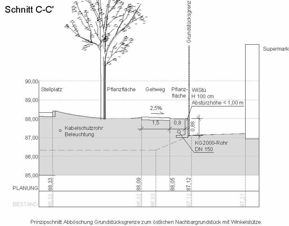
Schnitt C-C'
