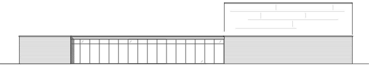
Ansicht Nord
