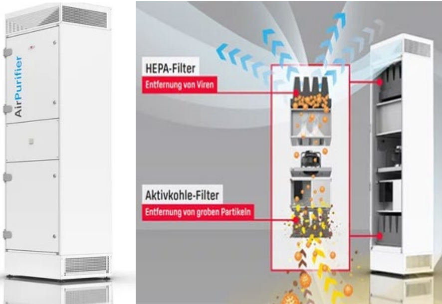
Filterbasiertes System
