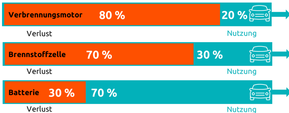
Abbildung 123: Vergleich Wirkungsgrad
