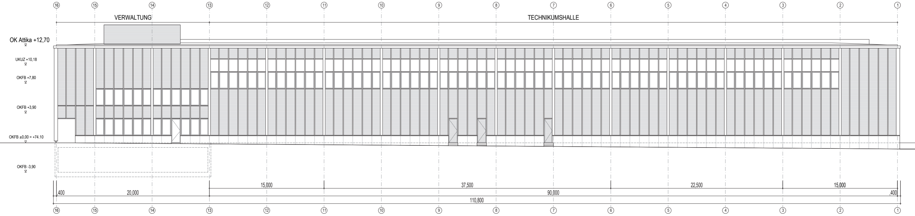
Ansicht West M 1:300
