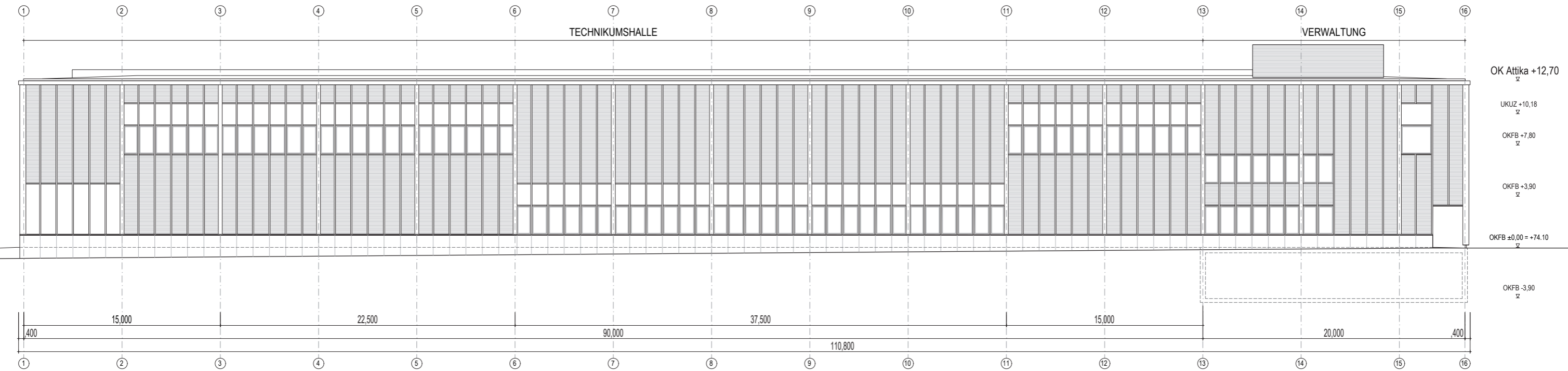
Ansicht Ost M 1:300
