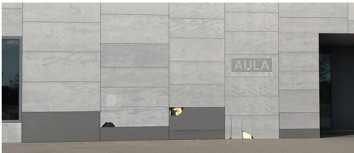
Neue Fassadenschäden – Fotos vom 17.10.2022
