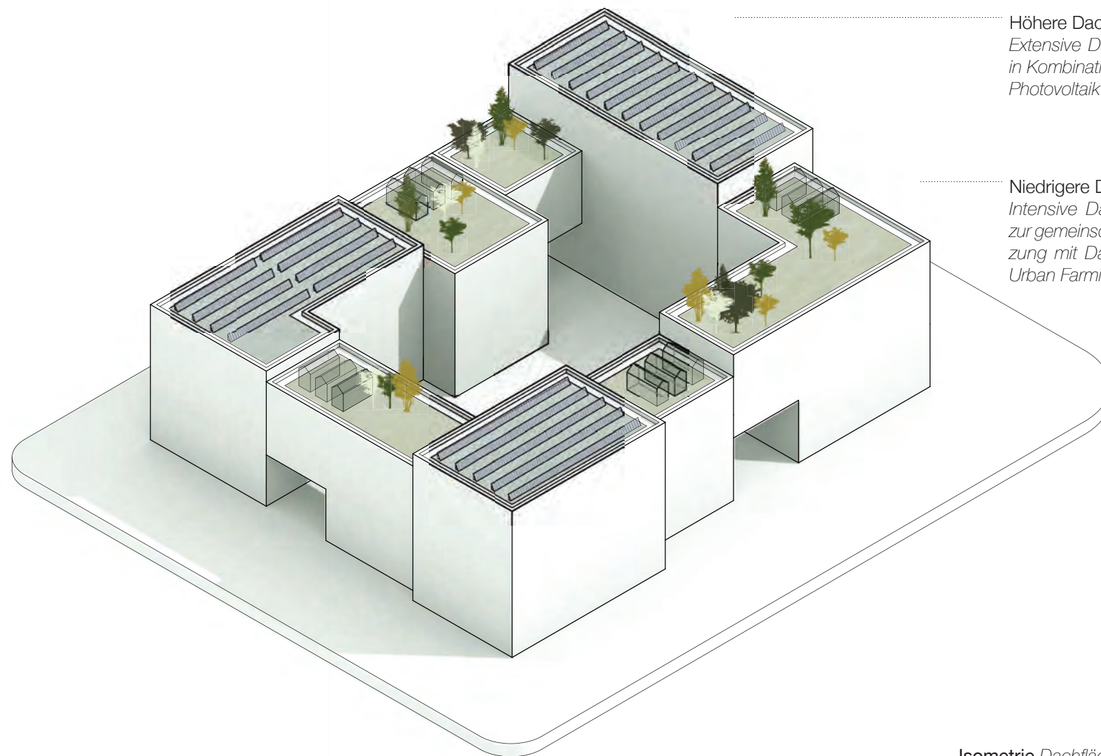
Isometrie Dachflächennutzungen
