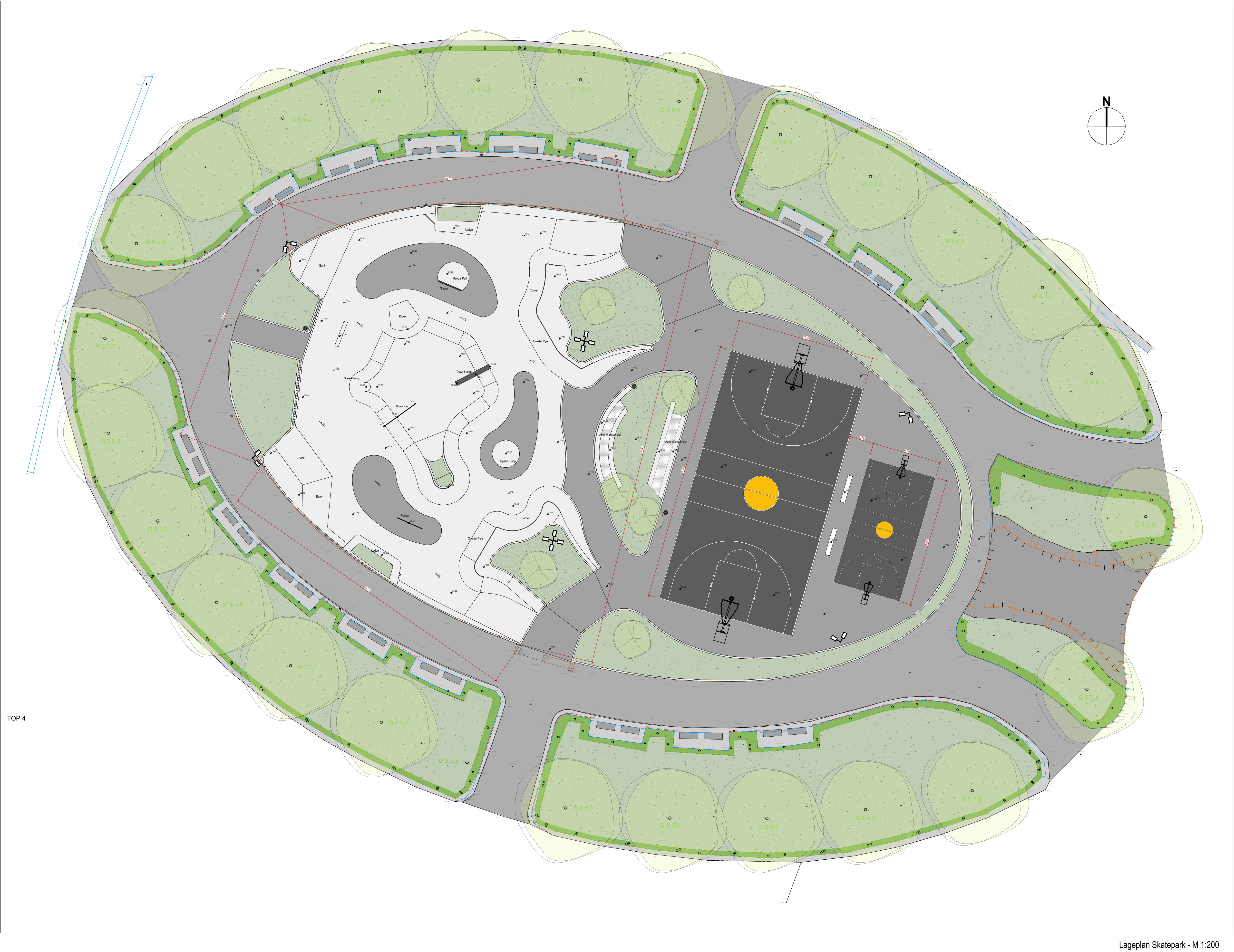
Lageplan Skatepark - M 1:200
