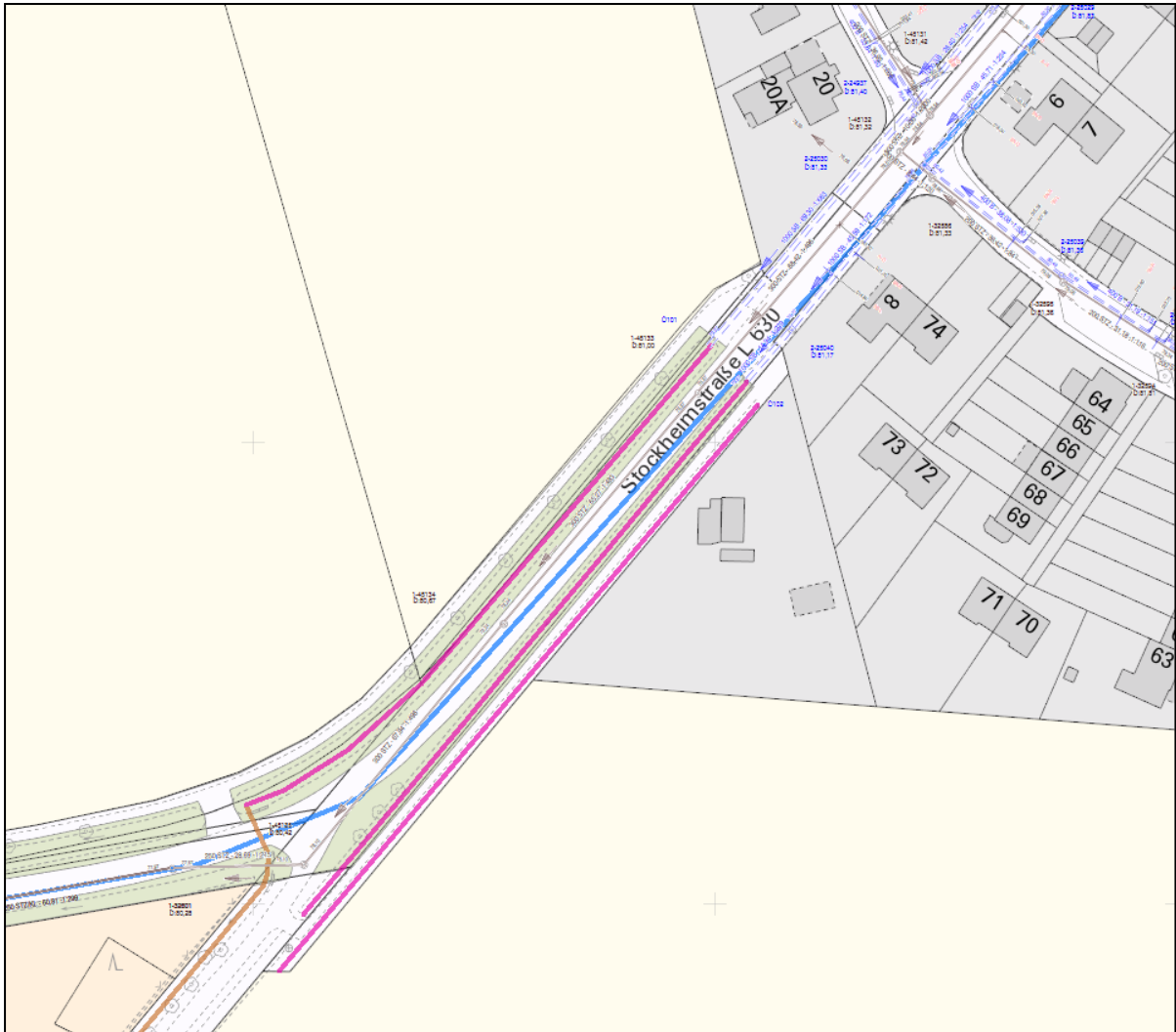
Abbildung 2: Lage der Einleitstellen O101 und O102 und der Regenwasserkanäle im Bereich der Stöckheimstraße
