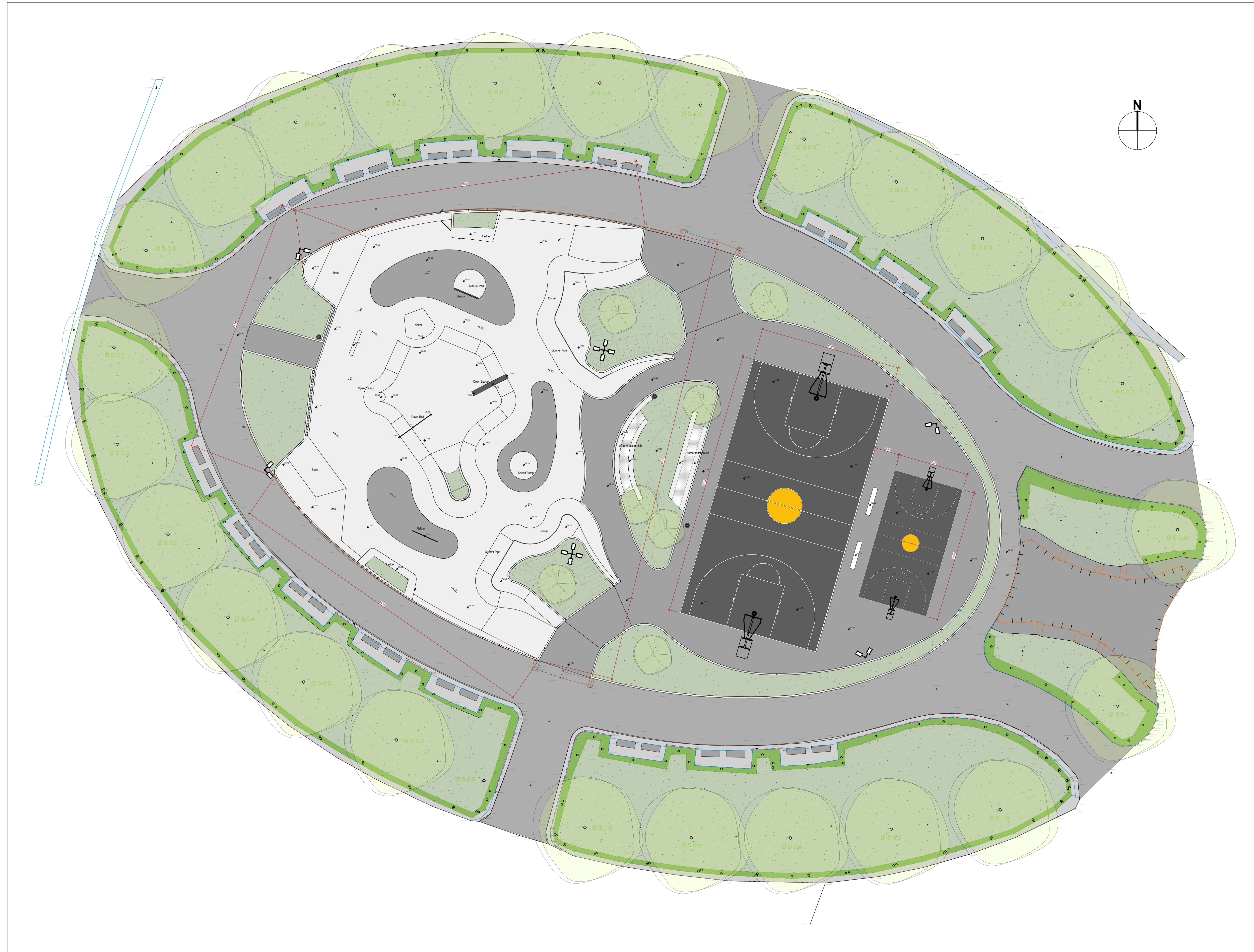
Lageplan Skatepark - M 1:200
