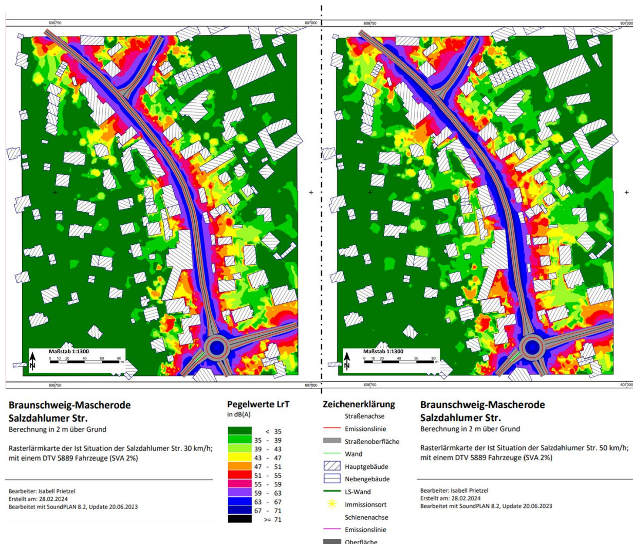
Abb. 24: Lärmberechnung des Untersuchungsgebietes für 30 km/h und 50 km/h (SoundPLAN) © Stadt Braunschweig I Abteilung Geoinformation (61.2/23-612-232)
